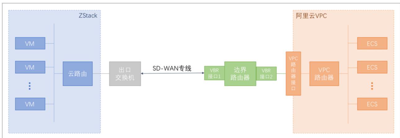
图 146: 大河高速通道网络架构图
