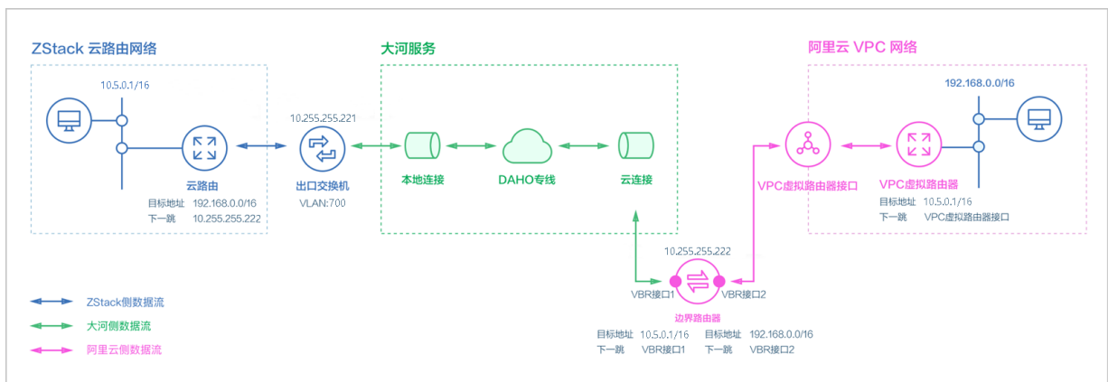
图 195: 大河高速通道网络拓扑图
