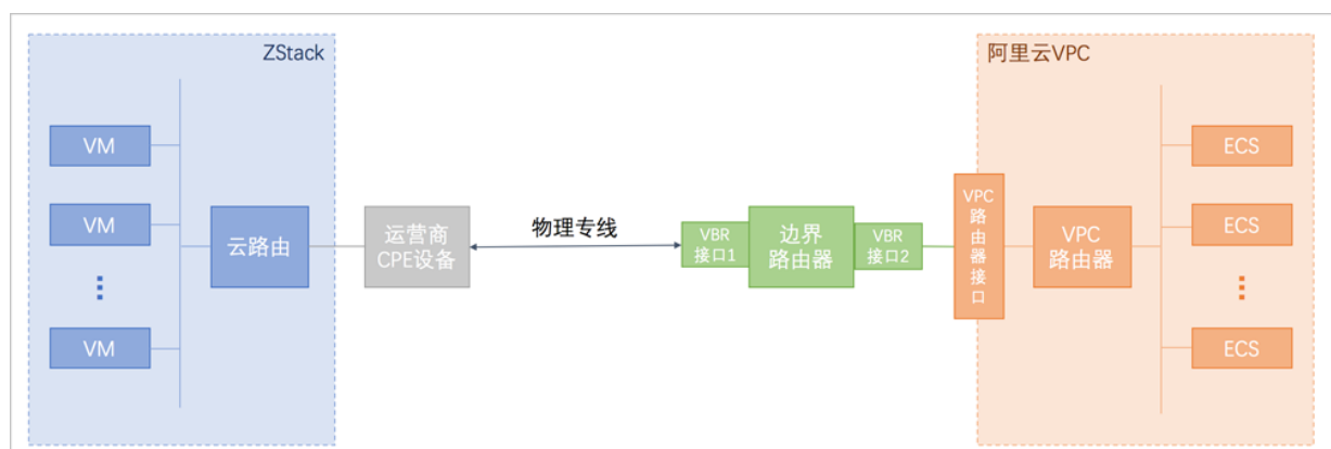
图 113: 阿里云高速通道网络架构图
