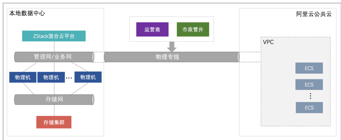
图 1: 基于物理专线部署
