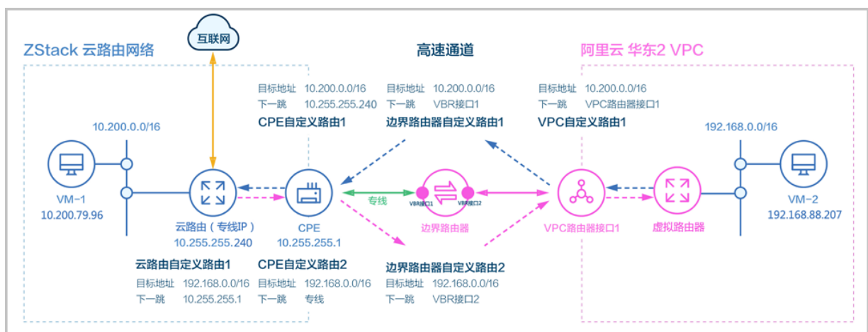
图 173: 高速通道网络架构图
