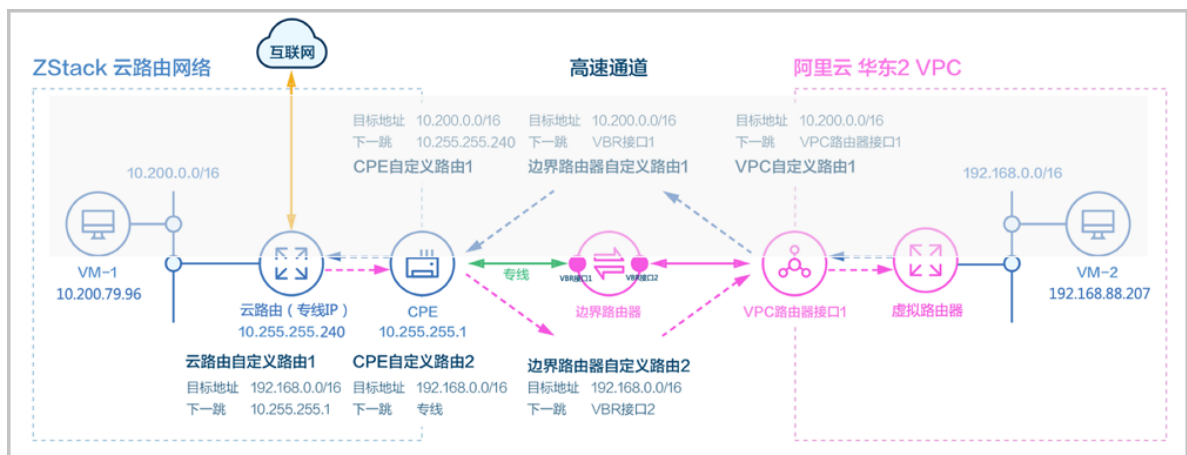
图 174: 本地云主机连通阿里云ECS的路由步骤
